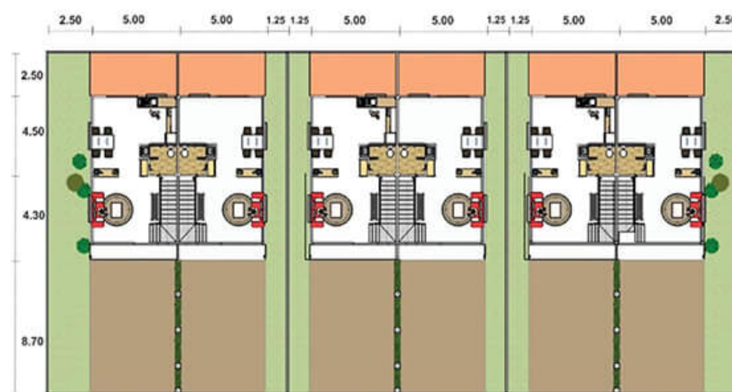
แปลนชั้น 1
